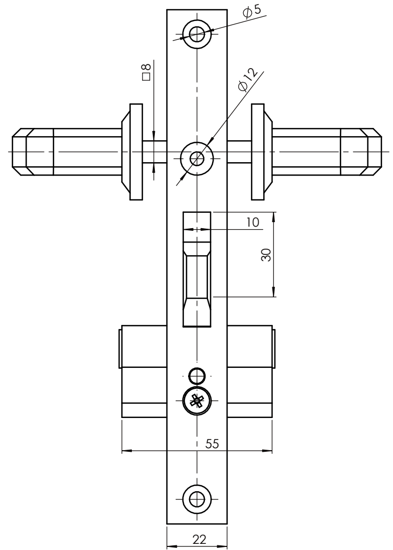
Ansicht ohne Stulp, Schlüssel und Schrauben
