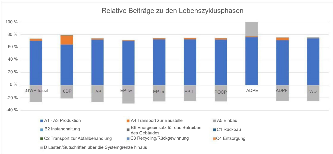
Abbildung 1: Umweltauswirkungen von Beschlägen für Schiebetüren über ihren Lebenszyklus
